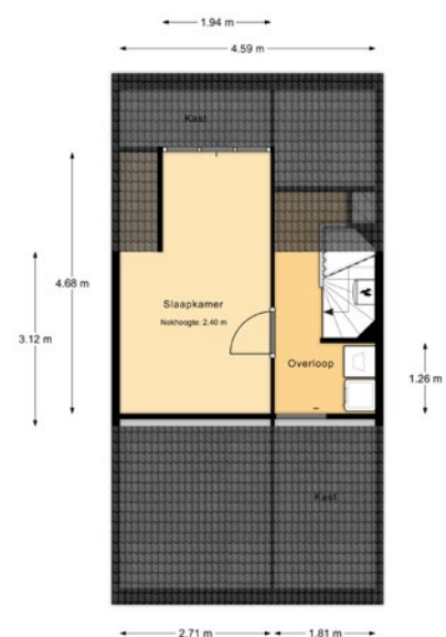
2e verdieping
