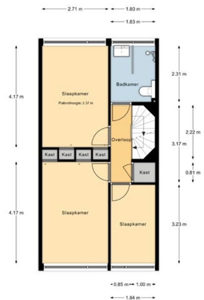
1e verdieping
